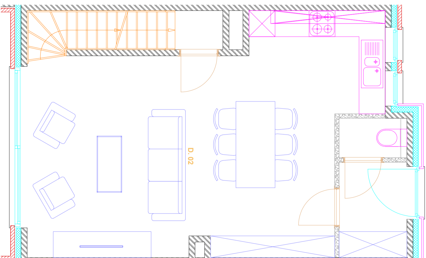
Gelijkvloers
